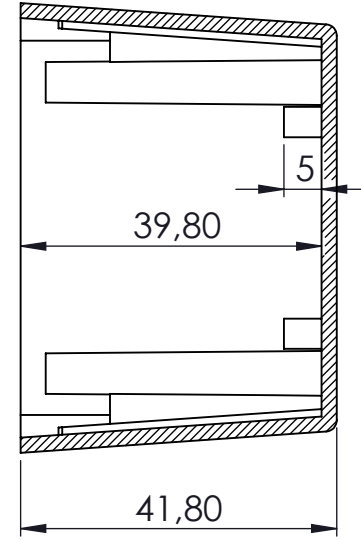
KESİT A-A
