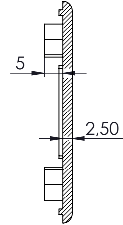
KESİT A-A
