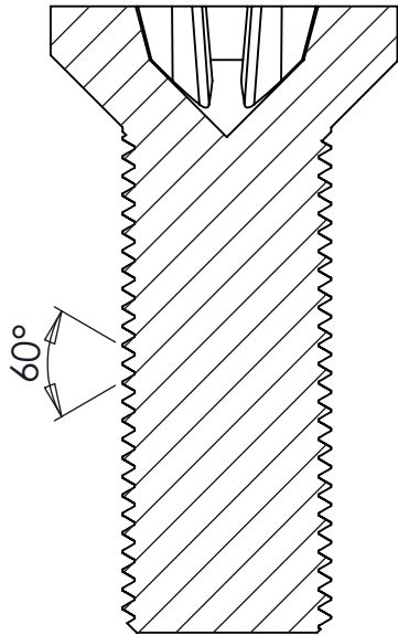
KESIT A-A
