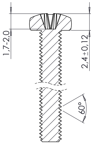
KESIT B-B
