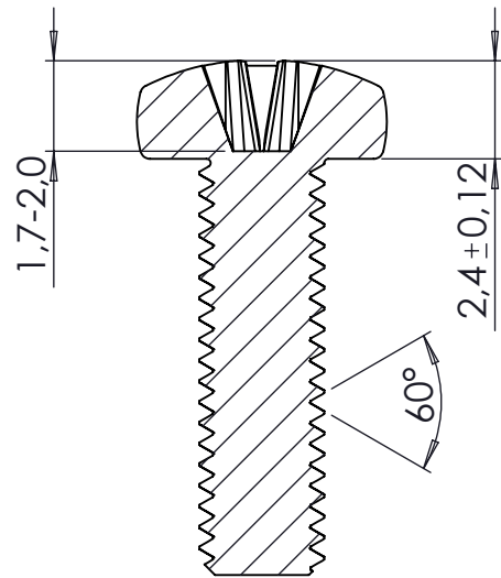
KESIT B-B
