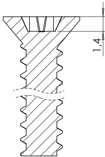
KESIT B-B
