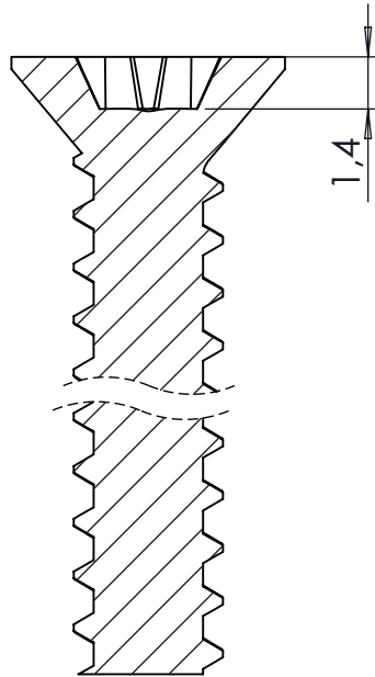
KESIT B-B
