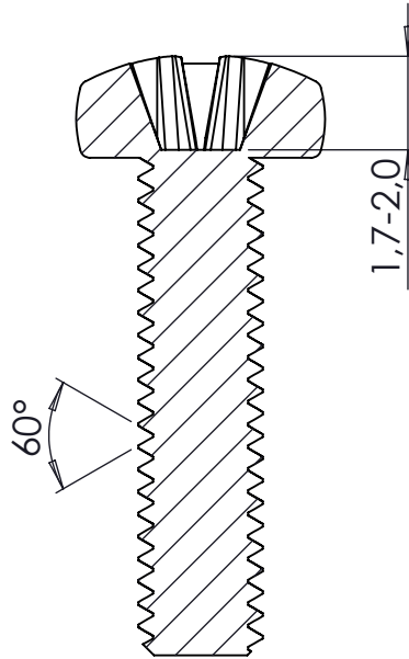
KESIT C-C
