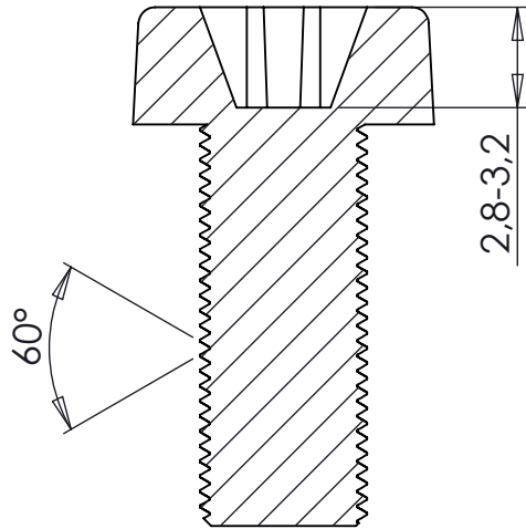
KESIT B-B
