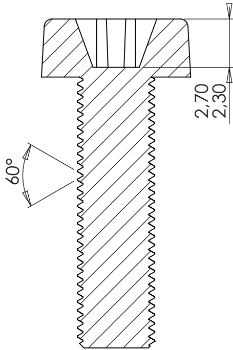
KESIT D-D
