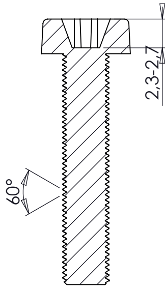
KESIT D-D
