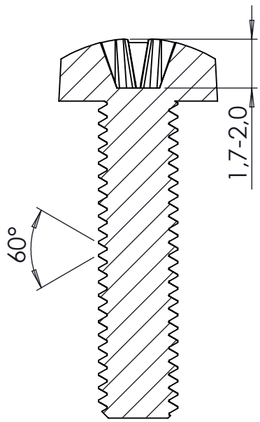
KESIT A-A
