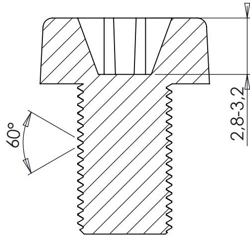
KESIT B-B
