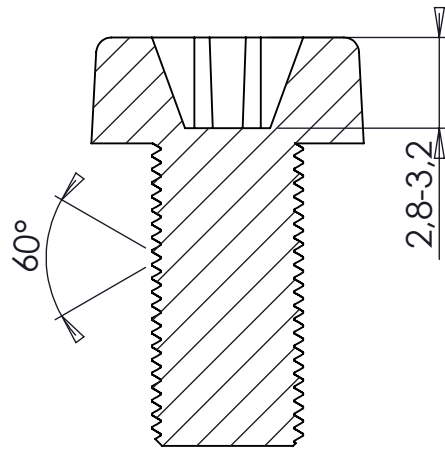
KESIT B-B
