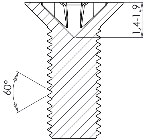
KESIT A-A
