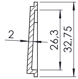
KESIT A-A
