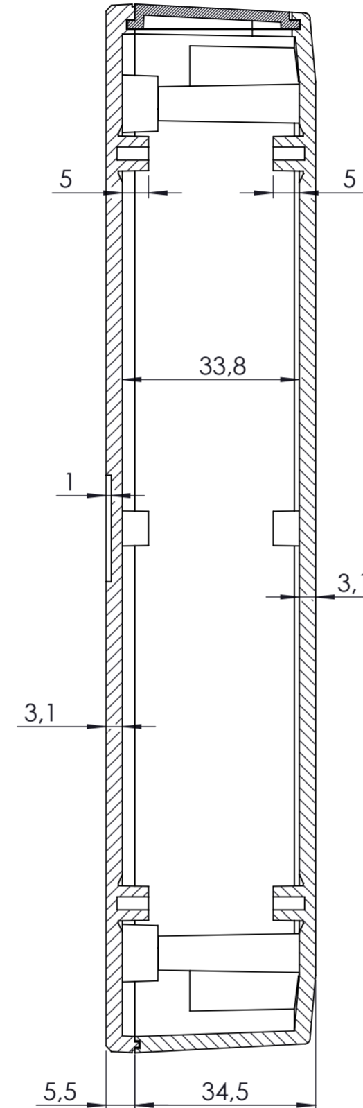
KESIT A-A
