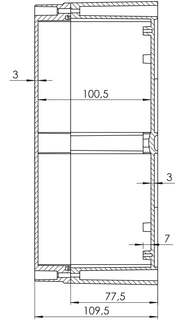
KESIT A-A
