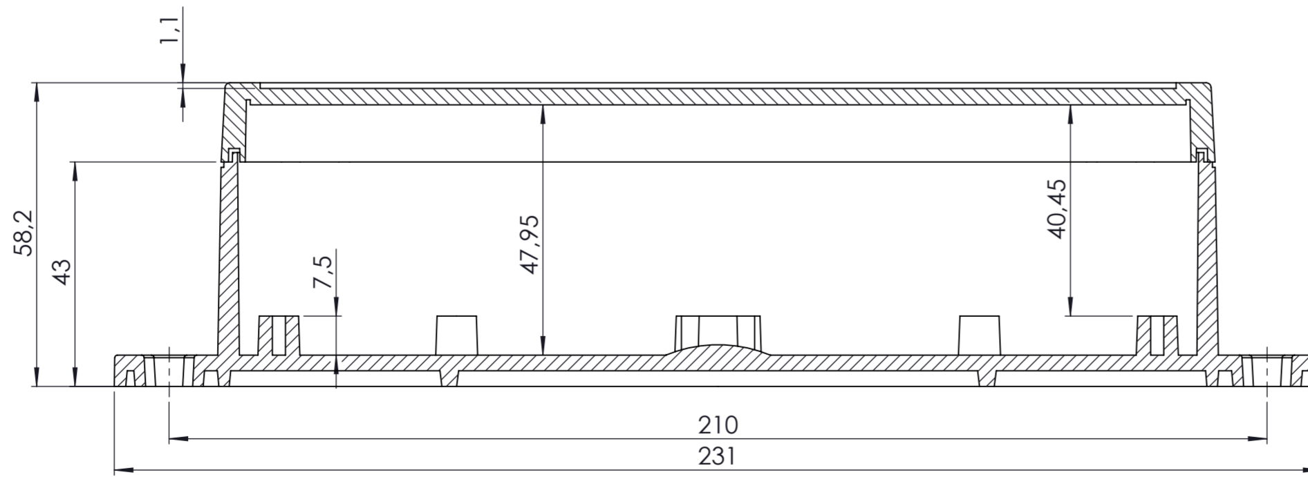
KESIT A-A
