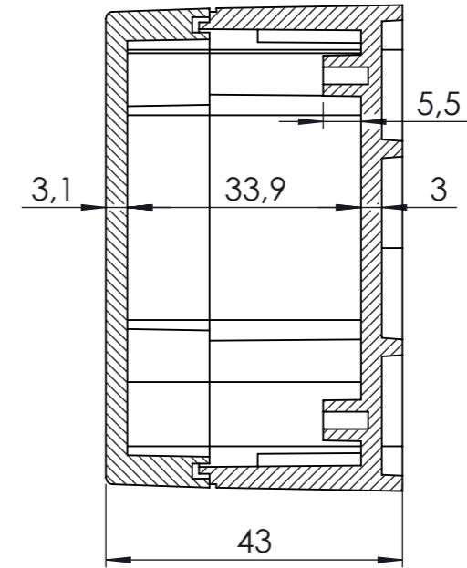
KESIT A-A
