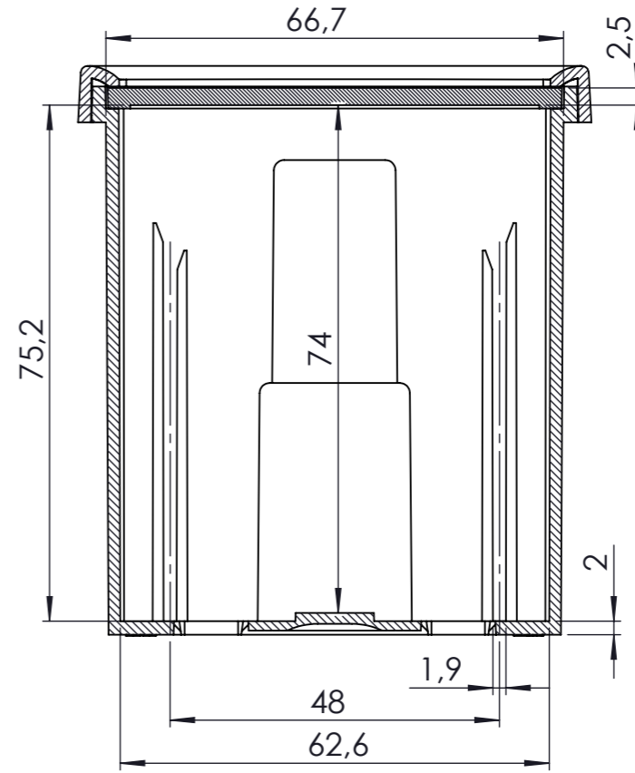
KESIT A-A
