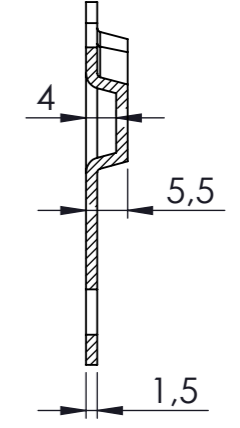
KESİT A-A
