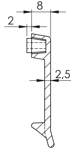
KESIT A-A
