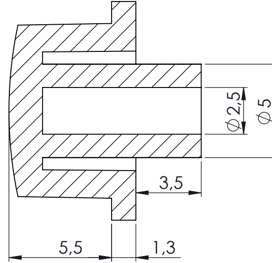
KESIT A-A
