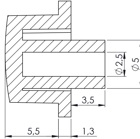
KESIT A-A
