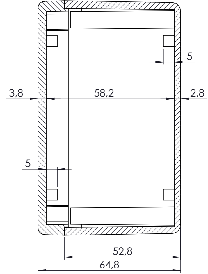
KESIT A-A
