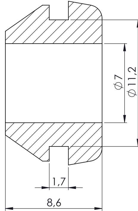
KESIT A-A
