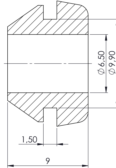
KESİT A-A
