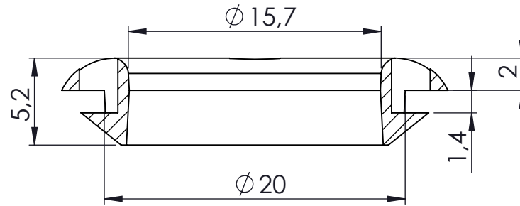
KESIT A-A
