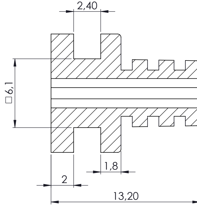
KESIT A-A
