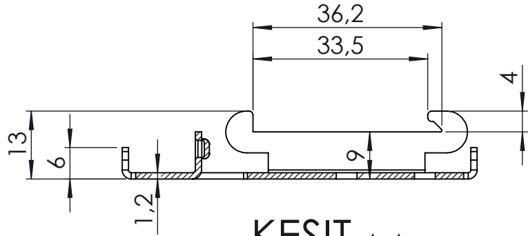
KESİT A-A
