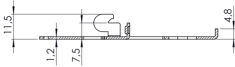
KESİT A-A
