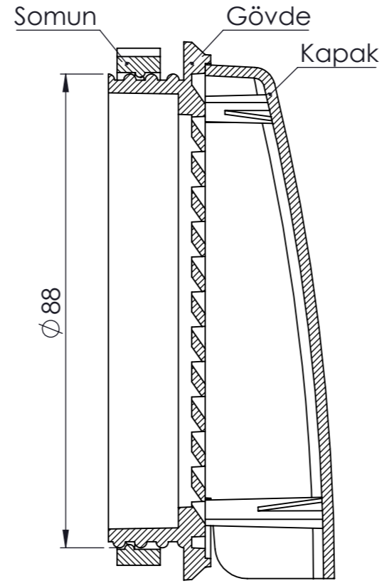
KESIT A-A
