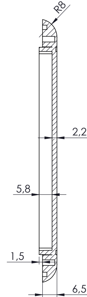
KESIT A-A
