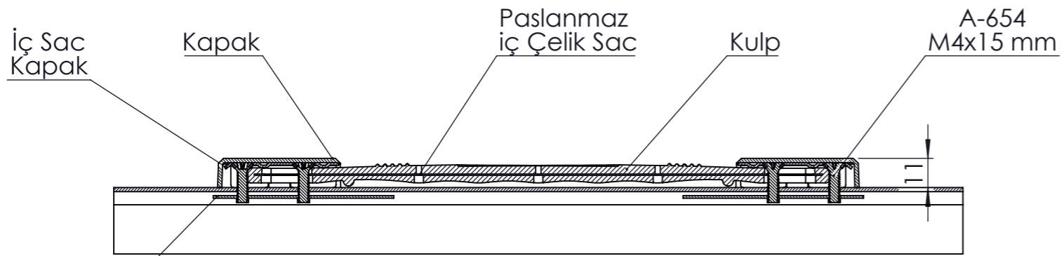
KESİT A-A
