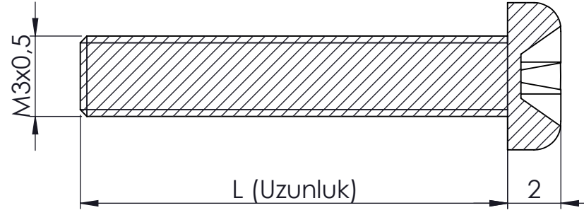
KESIT A-A
