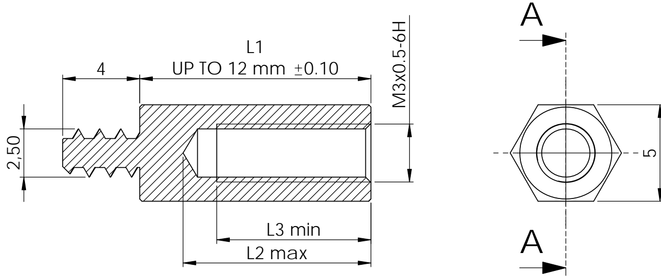
KESIT A-A
