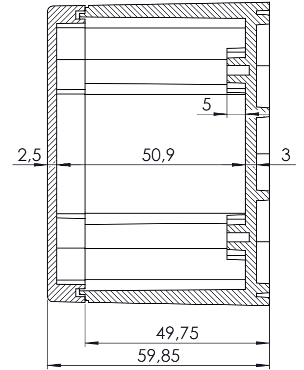
KESIT A-A
