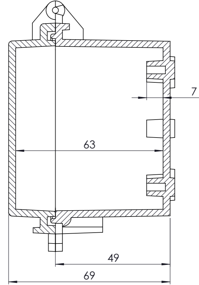
KESIT A-A
