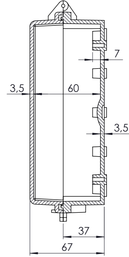
KESIT A-A
