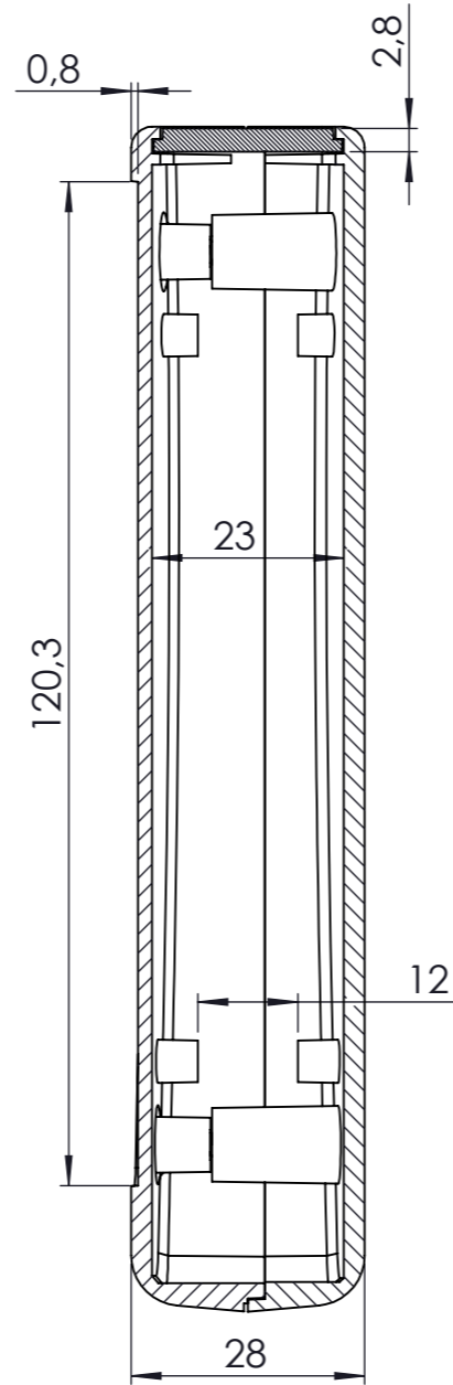
KESIT A-A
