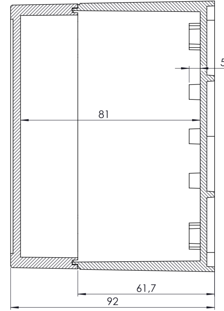
KESIT A-A
