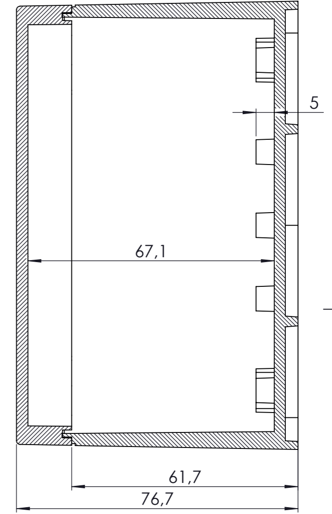
KESIT A-A
