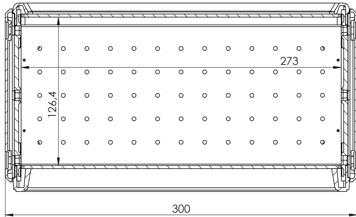
KESIT B-B
