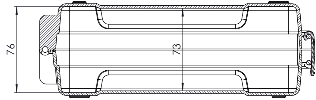
KESİT A-A
