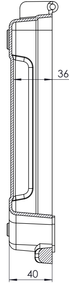
KESIT A-A
