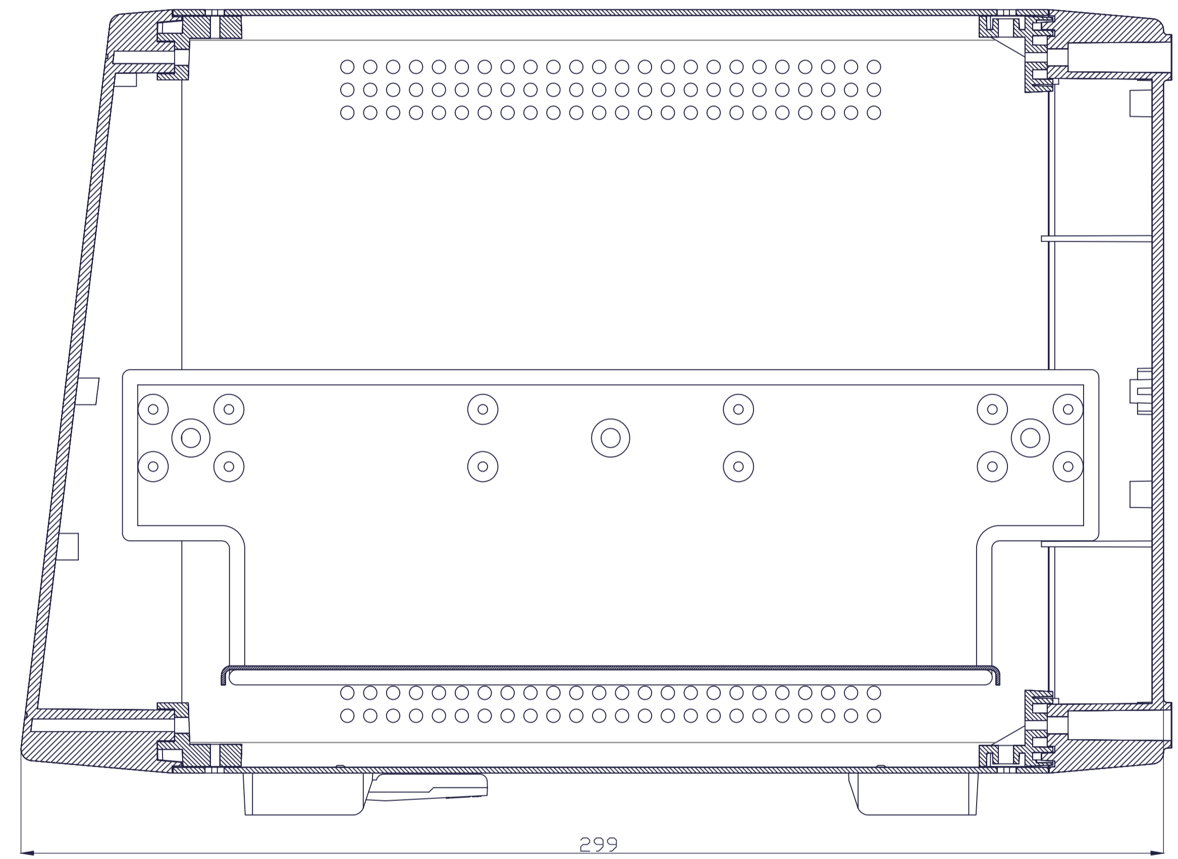
KESIT A-A
