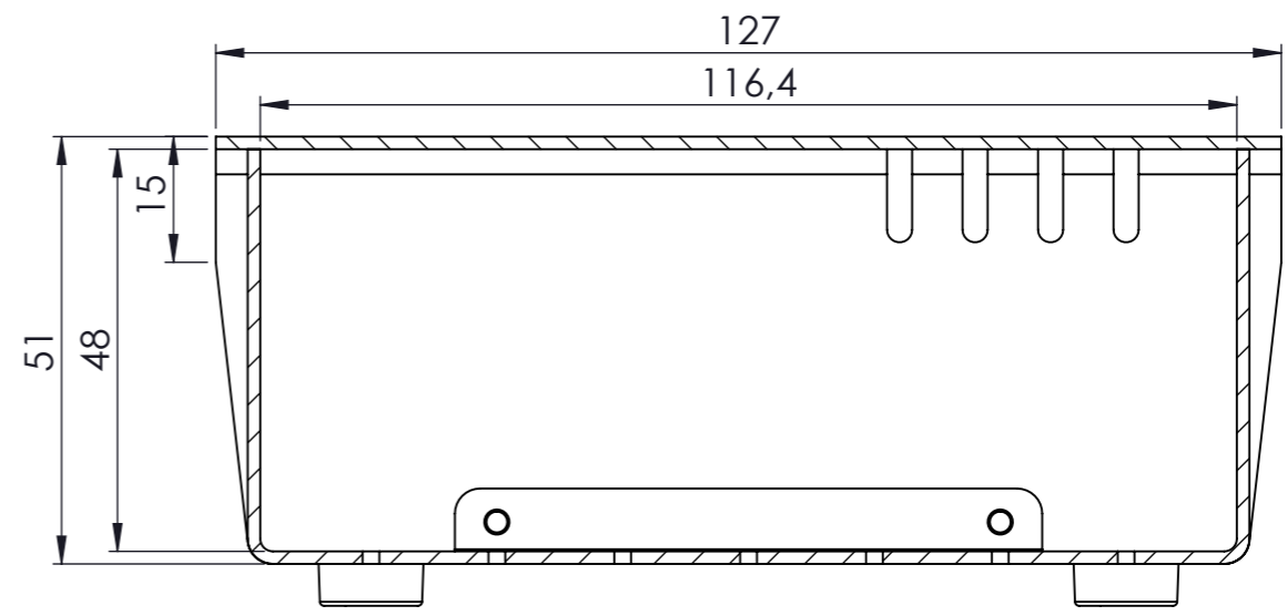
KESIT A-A
