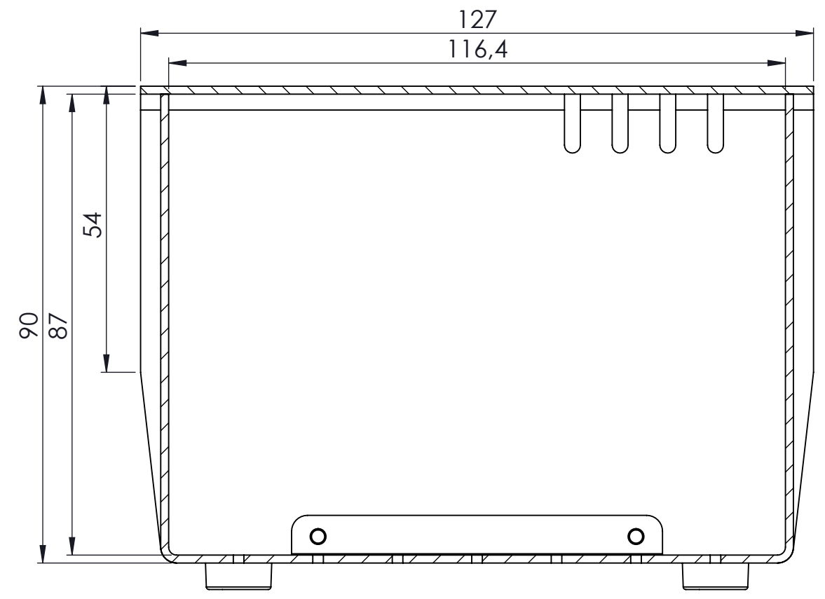
KESIT A-A
