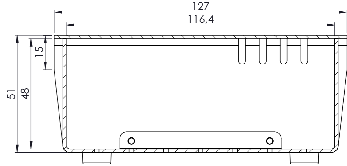
KESIT A-A
