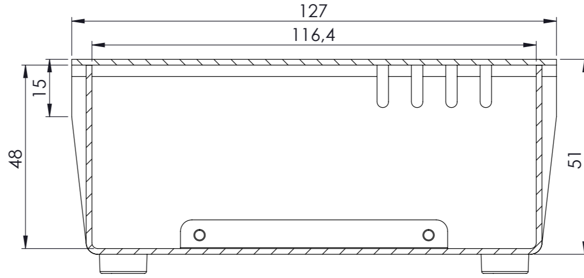
KESIT A-A
