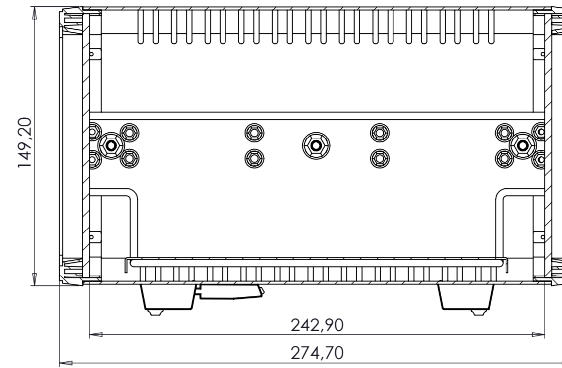
KESIT A-A
