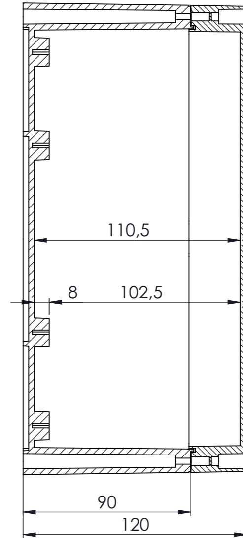
KESIT A-A
