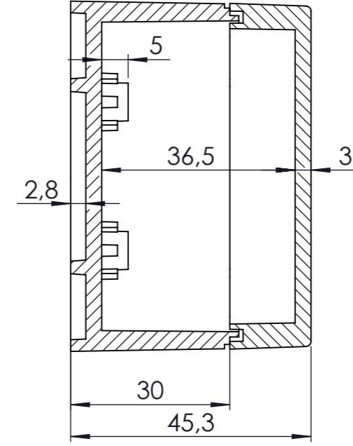
KESİT A-A
